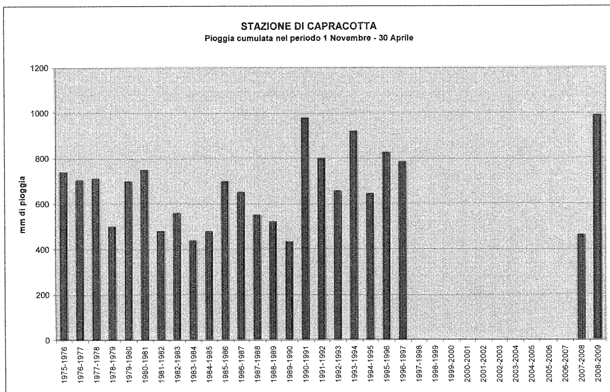
Figura 11: Precipitazioni cumulate 1 Novembre- 30 Aprile dal 1975 al 2009 - Stazione di Capracotta
