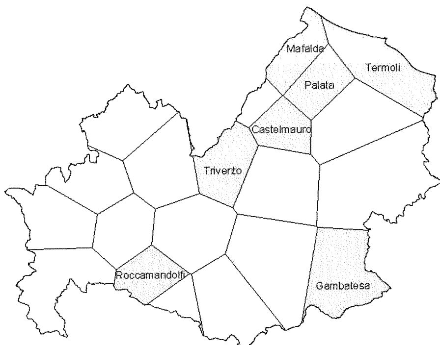
Figura 1: Area di influenza delle stazioni per cui è stato possibile ricostruire precipitazioni cumulate relative al periodo 1 Novembre–30 Aprile nell’arco degli ultimi 58 anni
