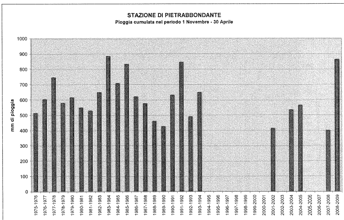
Figura 13: Precipitazioni cumulate 1 Novembre- 30 Aprile dal 1975 al 2009 - Stazione di Pietrabbondante
