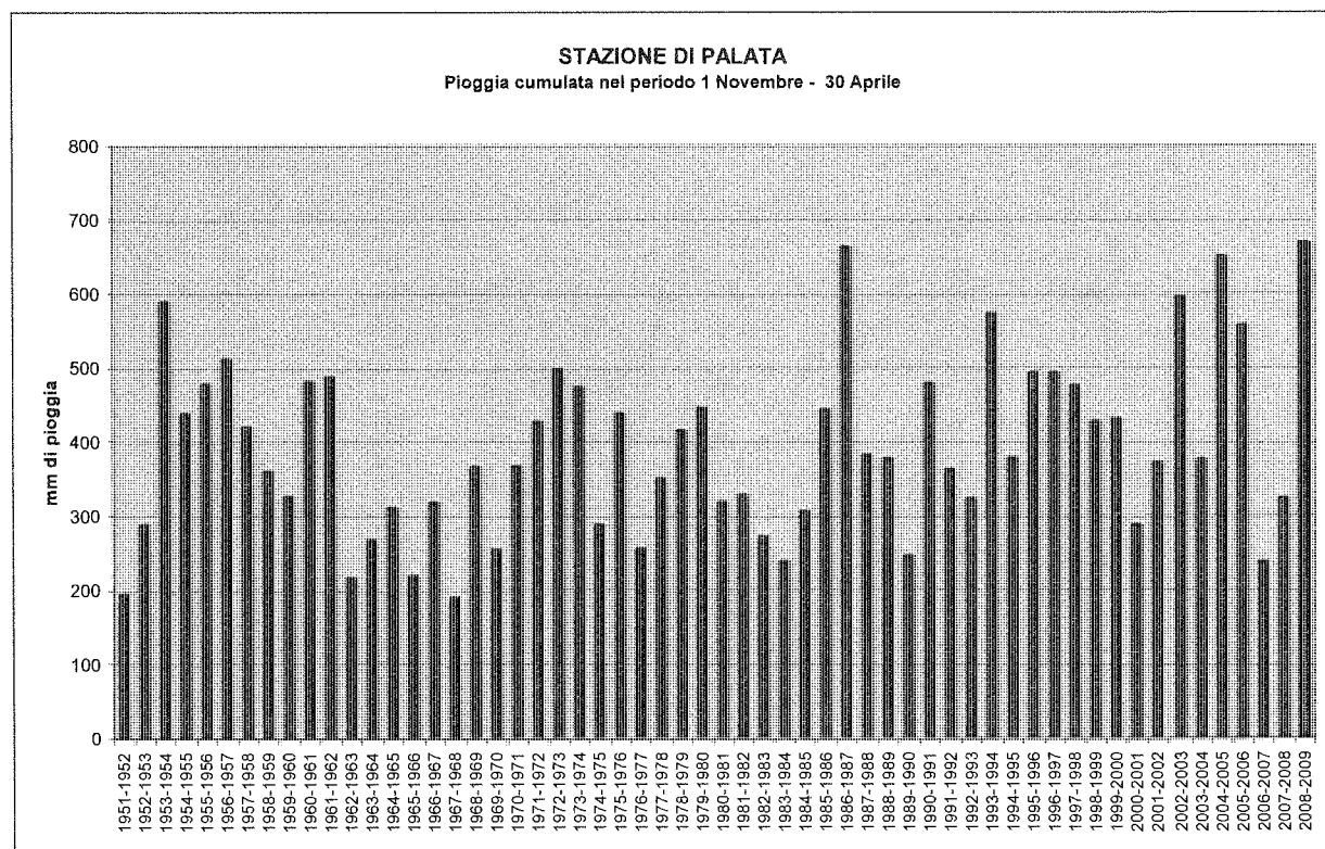
Figura 3: Precipitazioni cumulate 1 Novembre- 30 Aprile dal 1951 al 2009 - Stazione di Palata
