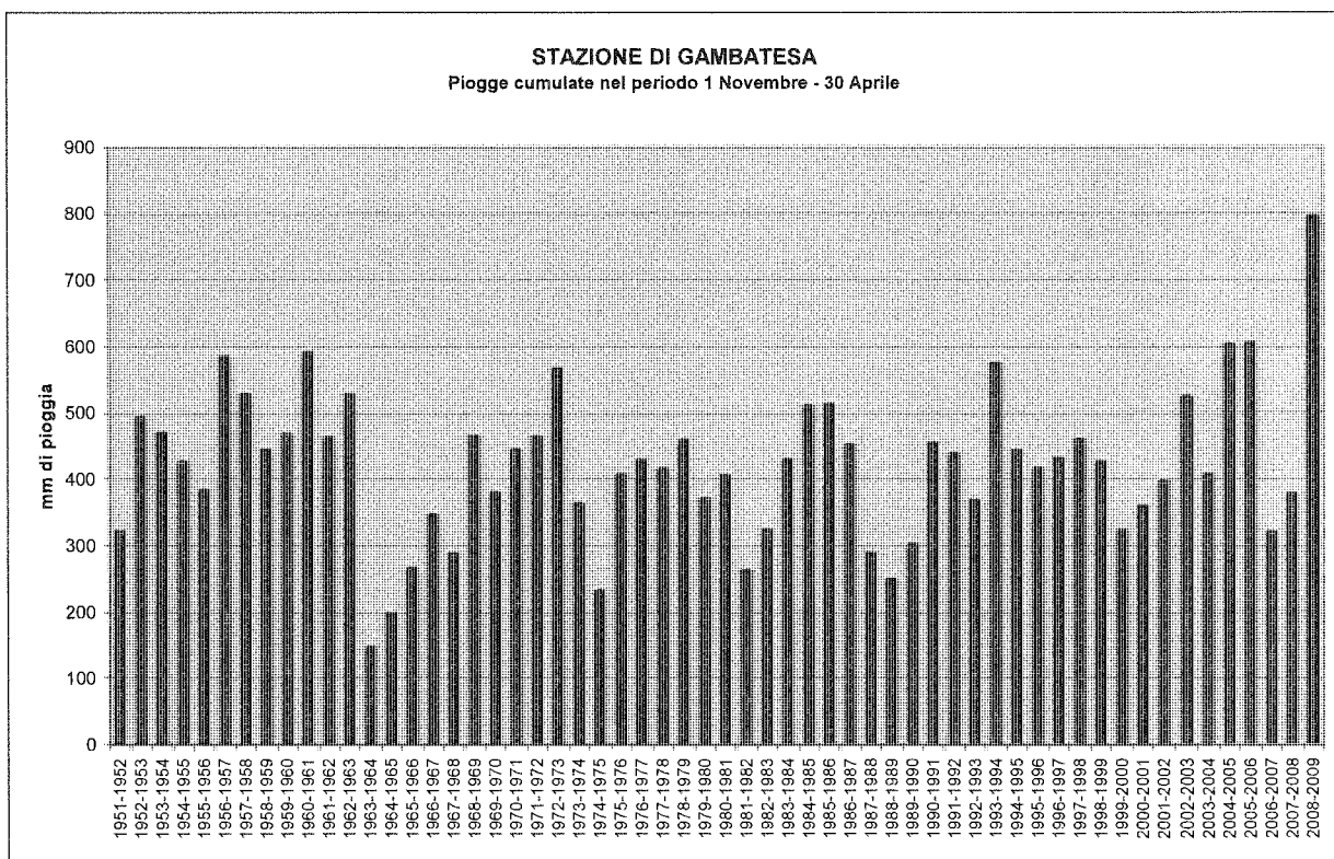
Figura 6: Precipitazioni cumulate 1 Novembre- 30 Aprile dal 1951 al 2009 - Stazione di Gambatesa
