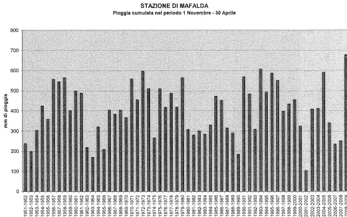
Figura 7: Precipitazioni cumulate 1 Novembre- 30 Aprile dal 1951 al 2009 - Stazione di Mafalda
