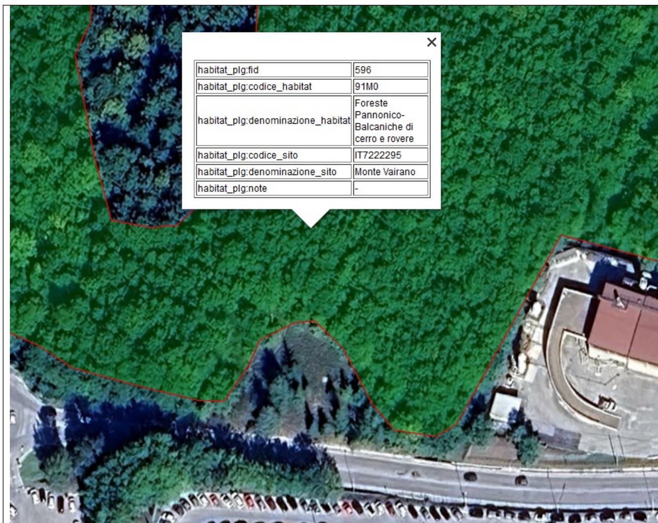
Planimetria 2) Area di intervento parzialmente collocata in sovrapposizione con habitat codice 91M0 "Foreste Pannonico-Balcaniche di cerro e rovere"
