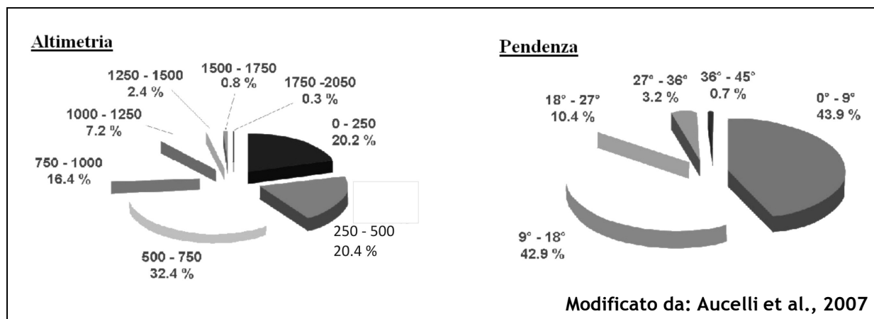
Figura 2 – Caratteristiche altimetriche e clivometriche del territorio molisano
