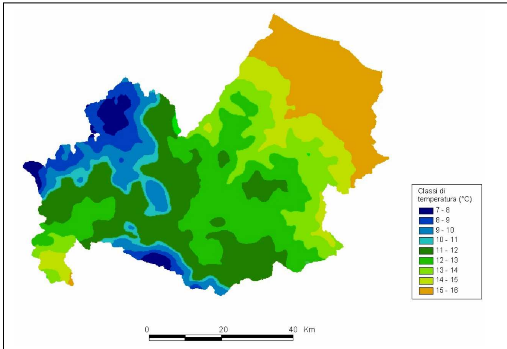
Figura 8 – Distribuzione delle temperature medie annue (in °C) in Molise (modificato da: Aucelli et al., 2007)
